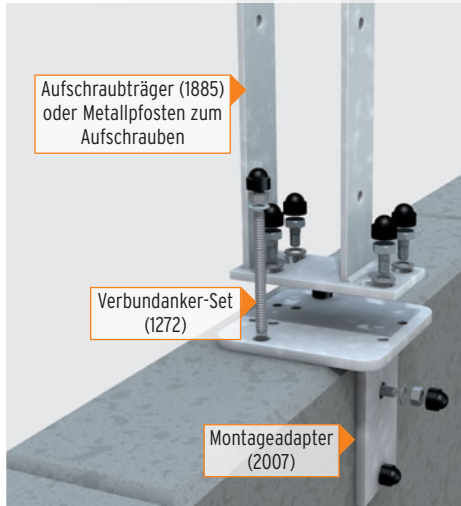
Aufschraubträger (1885) oder Metallpfosten zum Aufschrauben
