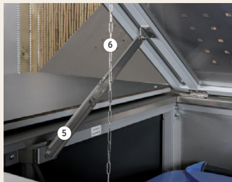
Variante met klapdeksel: Bediening met één hand door telescoop-opener (5) houdt het deksel open, trekking (6) opent het tonnendeksel "automatisch".
